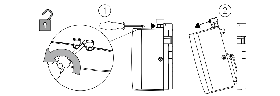
Fig. 13: « Dépose de l'appareil du support mural »
